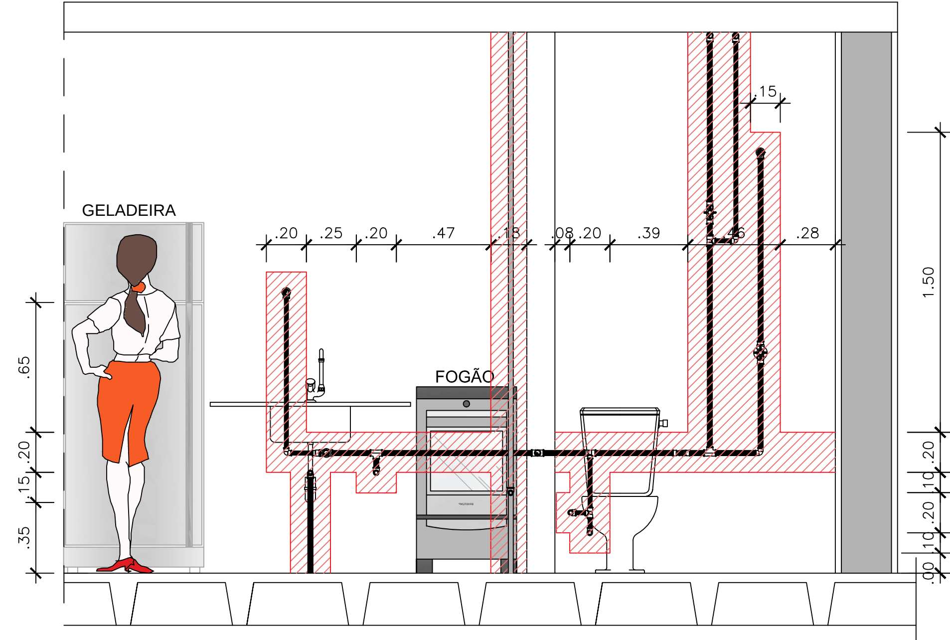
Vista J ESCALA 1/25
