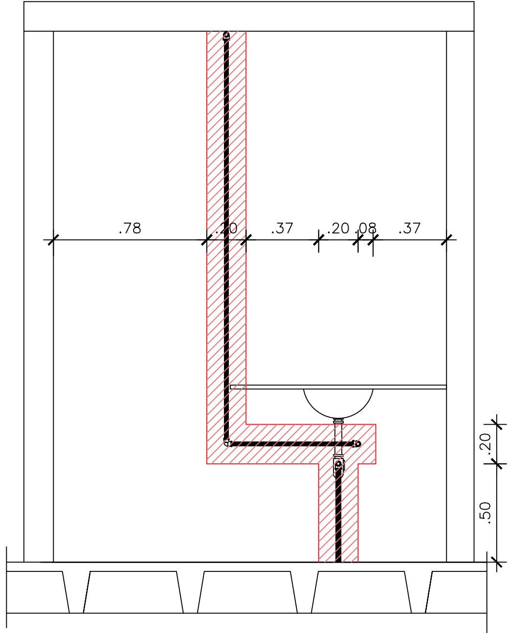
Vista I ESCALA 1/25
